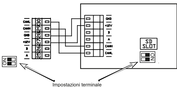
Collegamento elettrico
