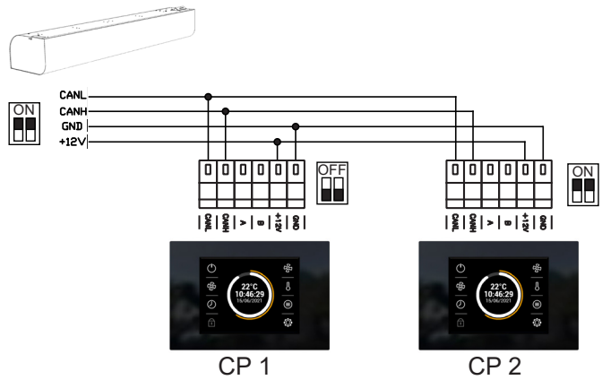
Conexión del cableado
