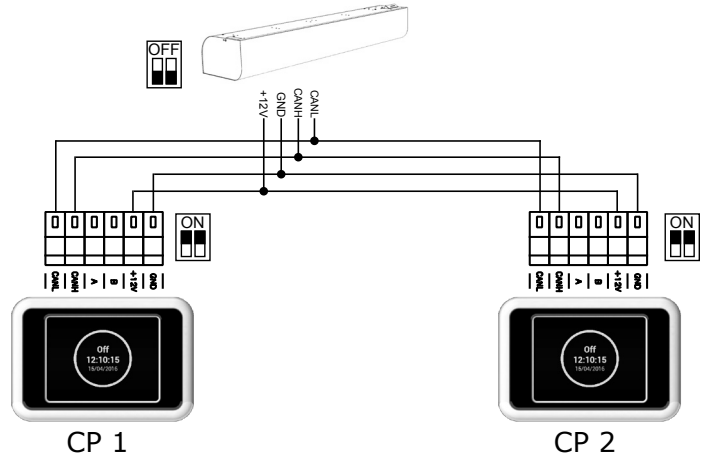
Collegamento elettrico - Opzione 2:
