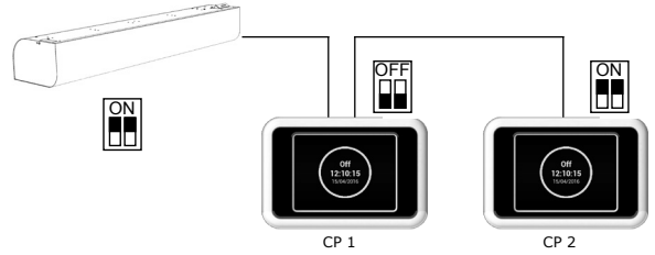
Collegamento elettrico - Opzione 1:
