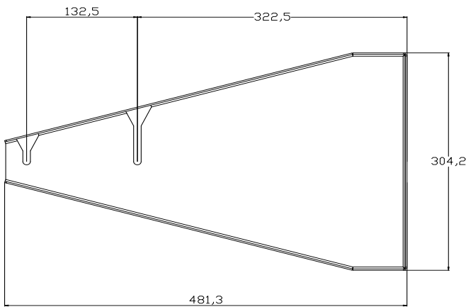
Schablone für die Positionierung der Savana-Wandhalterung
