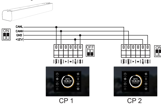
Elektrisk tilkobling
