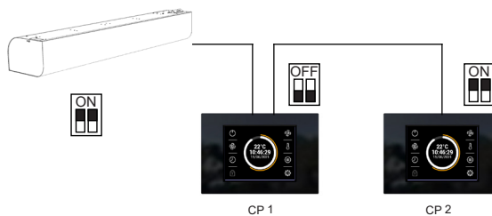
Elektrisk tilkobling
