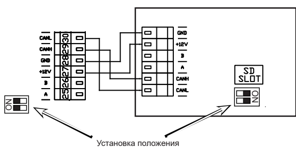
Электрическая схема подключения
