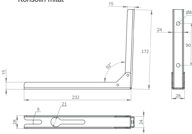
Konsolin mitat
