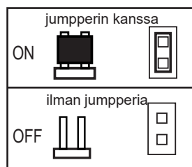
Jumpperin asento
