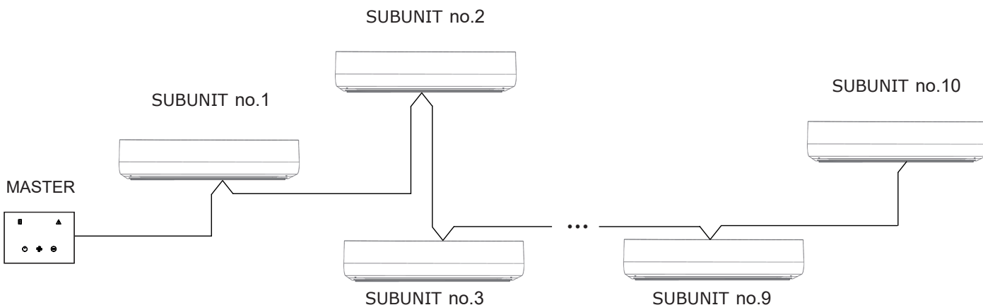
DIP asema
