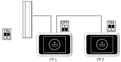
Collegamento elettrico - Opzione 1:
