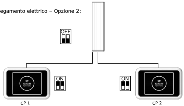
Collegamento elettrico - Opzione 2:
