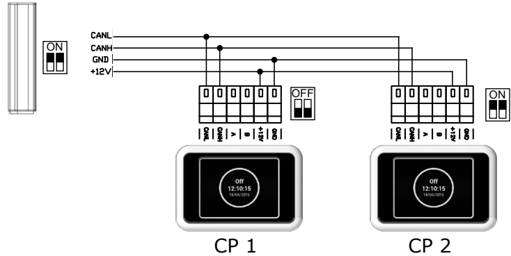
Collegamento elettrico - Opzione 1:
