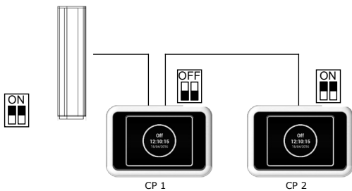
Collegamento elettrico - Opzione 1:
